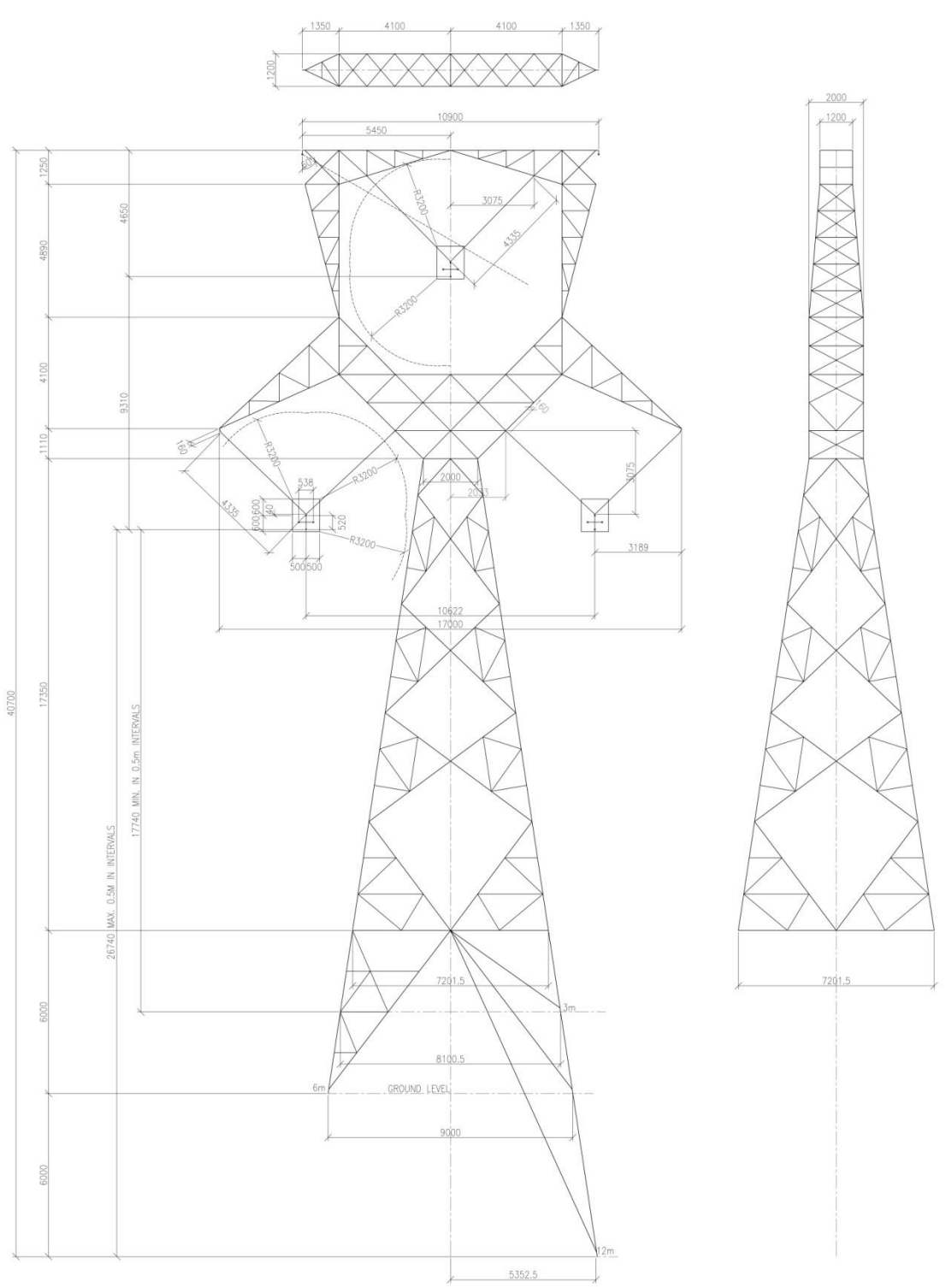
518E OUTLINE
